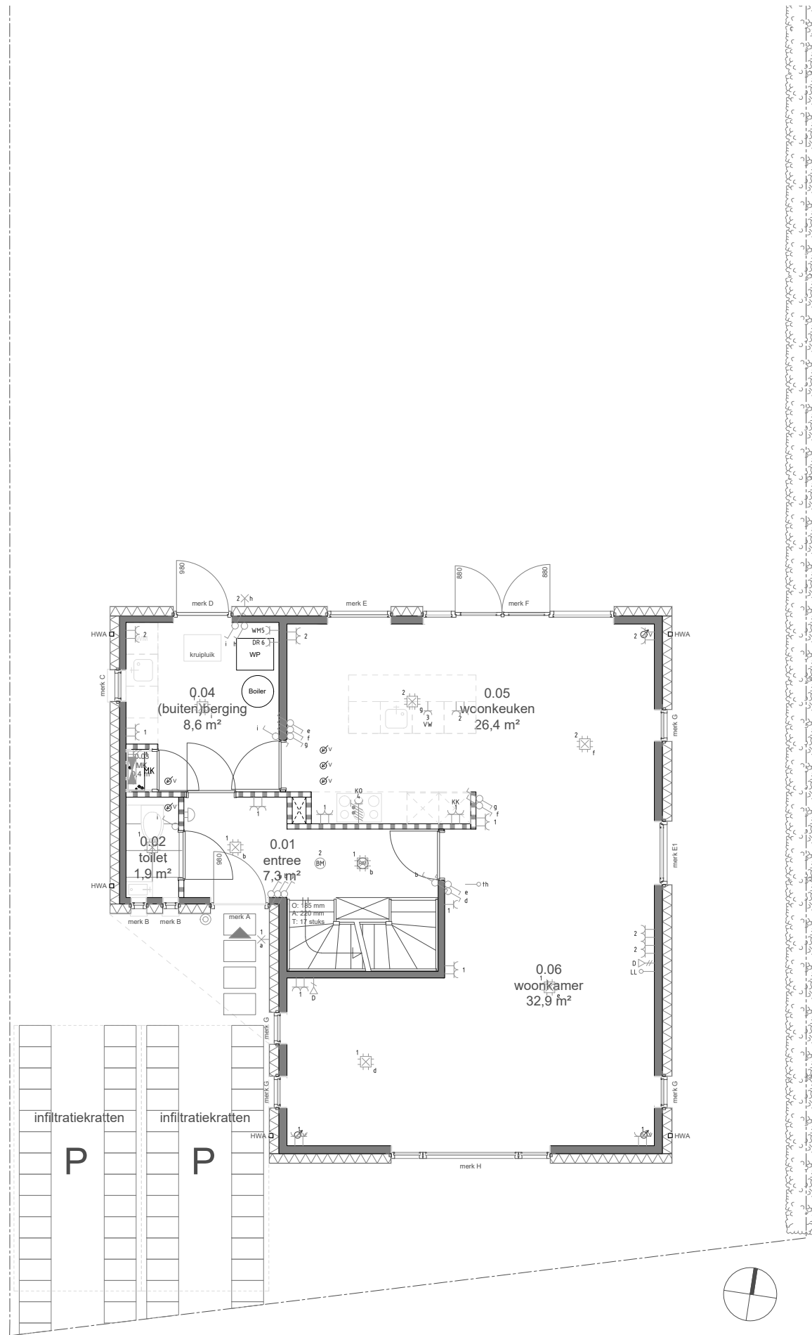
Begane grond
