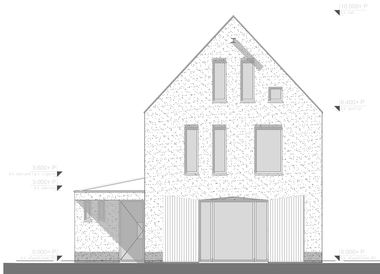
Voorgevel (zuid)
