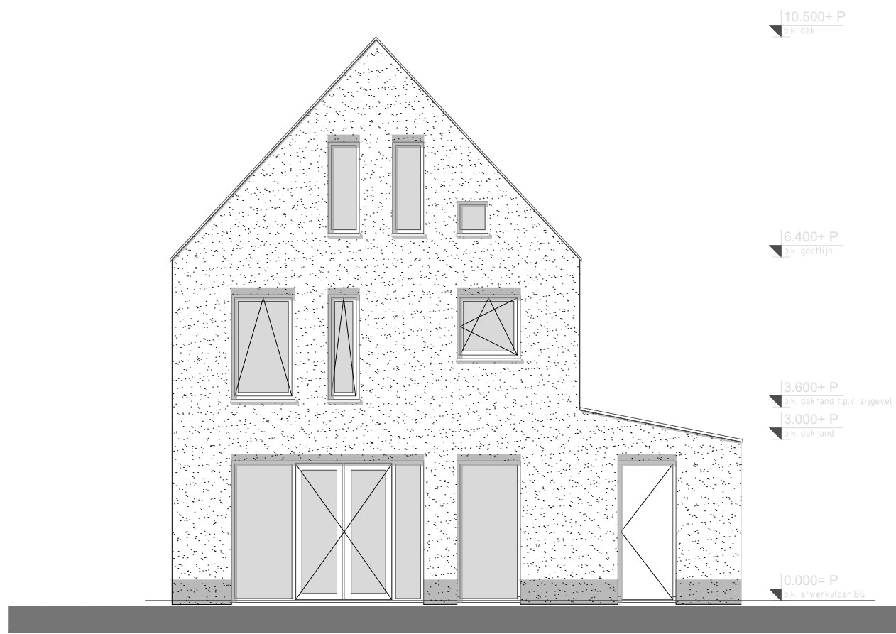
Achtergevel (noord)
